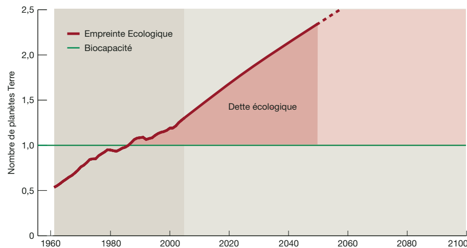
Fig. 31 : SCENARIO « BUSINESS AS USUAL » ET DETTE ECOLOGIQUE
